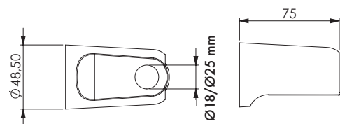
Supporto laterale fisso ABS cromato Ø 18 mm Fixed chromed ABS side bracket Ø 18 mm
