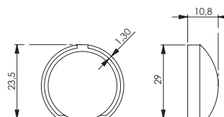
Placchetta grigia per supporto laterale per saliscendi Ø 18 mm e Ø 25 mm Grey plate for lateral bracket for sliding rails Ø 18 mm and 25 mm
